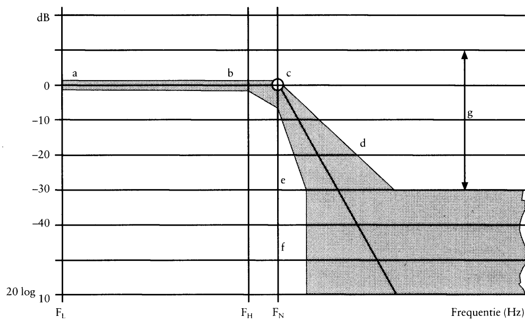
Frequentie-responsiekromme
